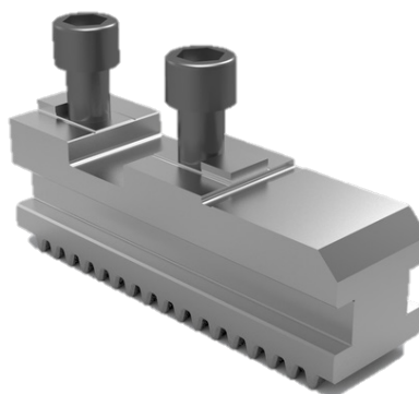
GRUNDBACKE FGB315
