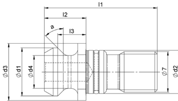
Anzugsbolzen DIN ISO 7388-3 UF (ISO 7388-2 Form B)
