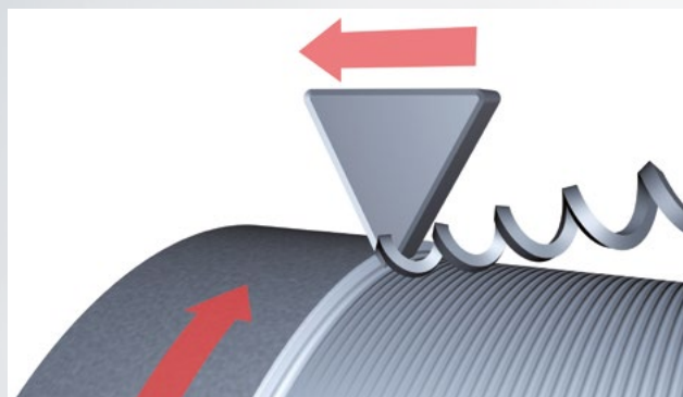
Drehvorgang / Turning process
