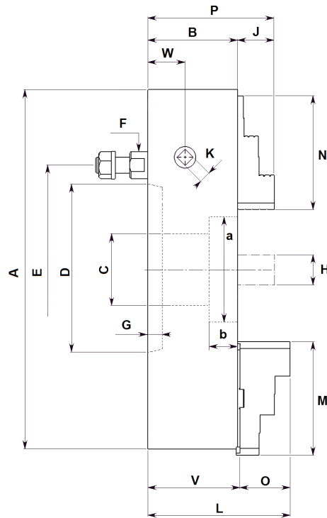
Maßtabellen für Drehfutter Type ADR/4
