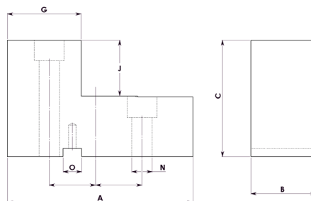
Gehärtete Aufsatzbacken Hardened top jaws Mors durs rapportés
