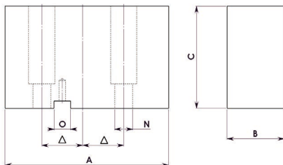
Weiche Aufsatzbacken Soft top jaws RD Mors doux rapportés
