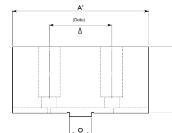
Weiche Aufsatzbacken Soft top jaws Mors doux rapportés
