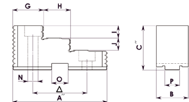
Gehärtete Aufsatzbacken (A' + C') Hardened top jaws Mors durs rapportés
