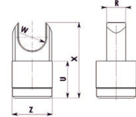
Haltebolzen Nut Support de vis
