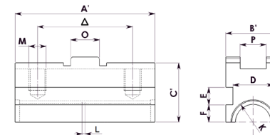
Gehärtete Grundbacken Hardened base jaws Semelles trempées
