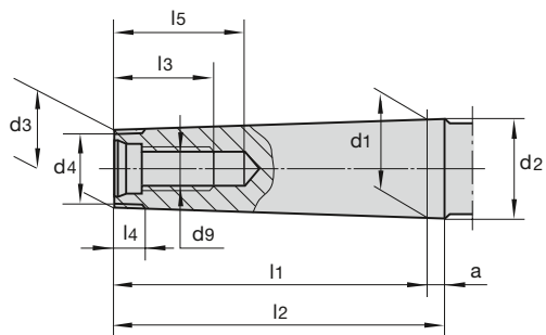
DIN 228 A
