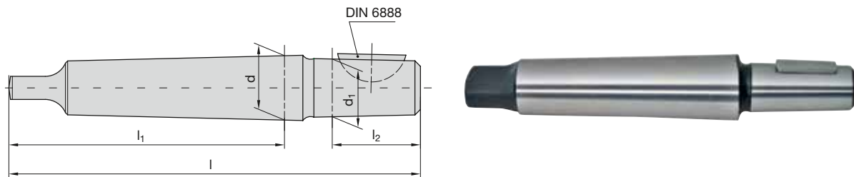
Kegelhorn DIN 238 mit Scheibenfeder DIN 6888 Arbor DIN 238 with woodruff key DIN 6888
